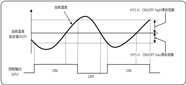
[图25] ON/OFF控制
