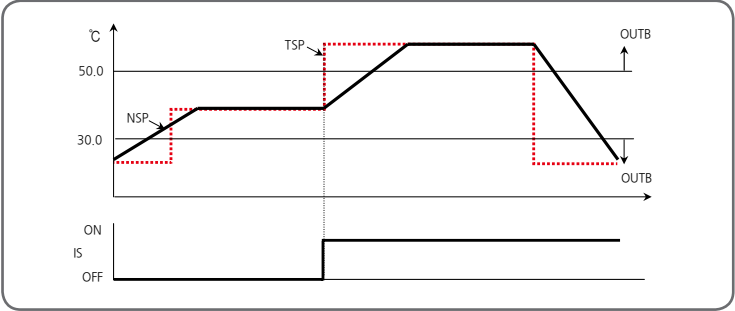
[图32] 内部信号动作例 #4
