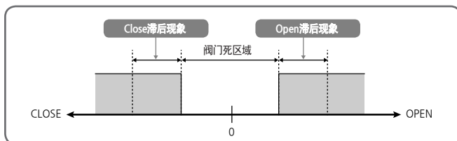
[图23] V.DB、V.HYS 操作
