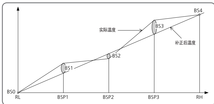
[图17] 区间别输入补正(BIAS)设定例
