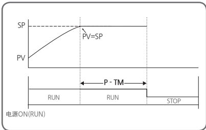
[图14] PV=SP模式动作
