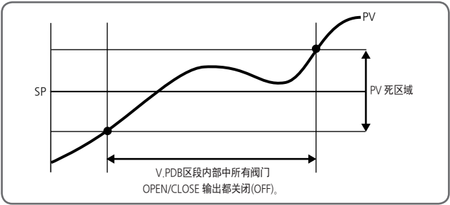
[图24] V.PDB(阀门PV死区域)
