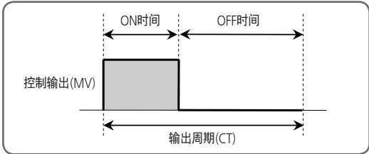
[图39] 取暖器断线警报检测条件
