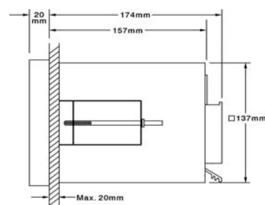
圖 2-3 盤面開孔(標準 DIN 尺寸 138mm x 138 mm)
