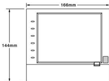
圖 2-1 正面圖
