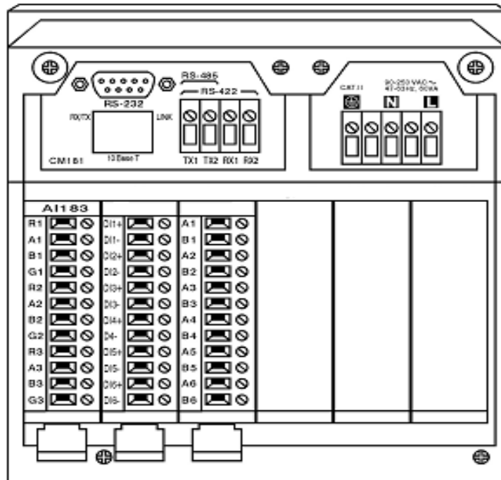
圖 2-17 記錄器後側端子圖
